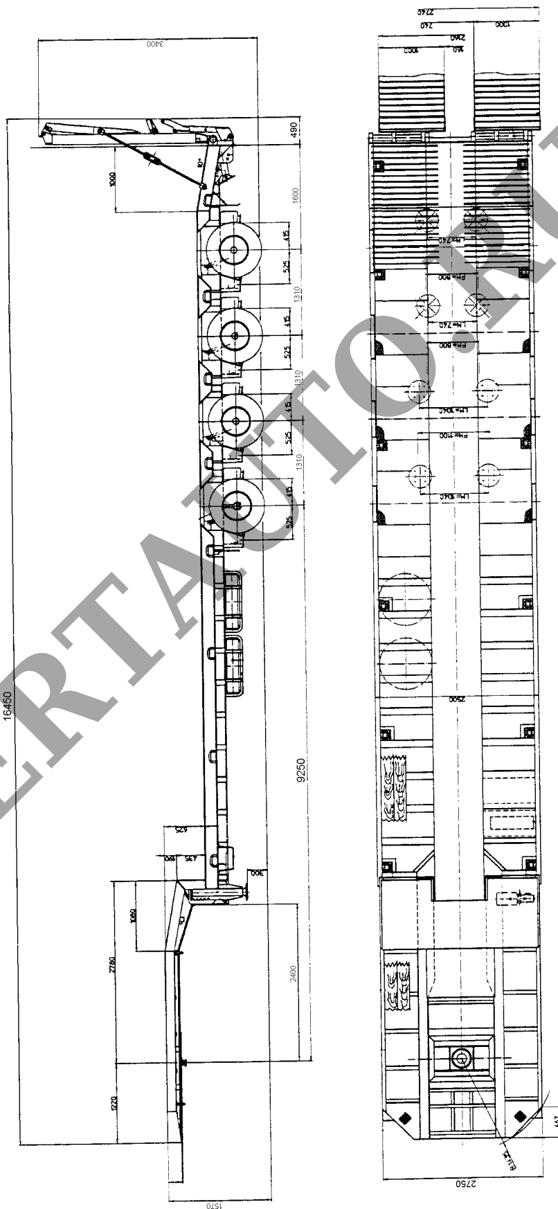
Рис.1. Полуприцеп GOLDHOFER модели STN-L4-56/60
