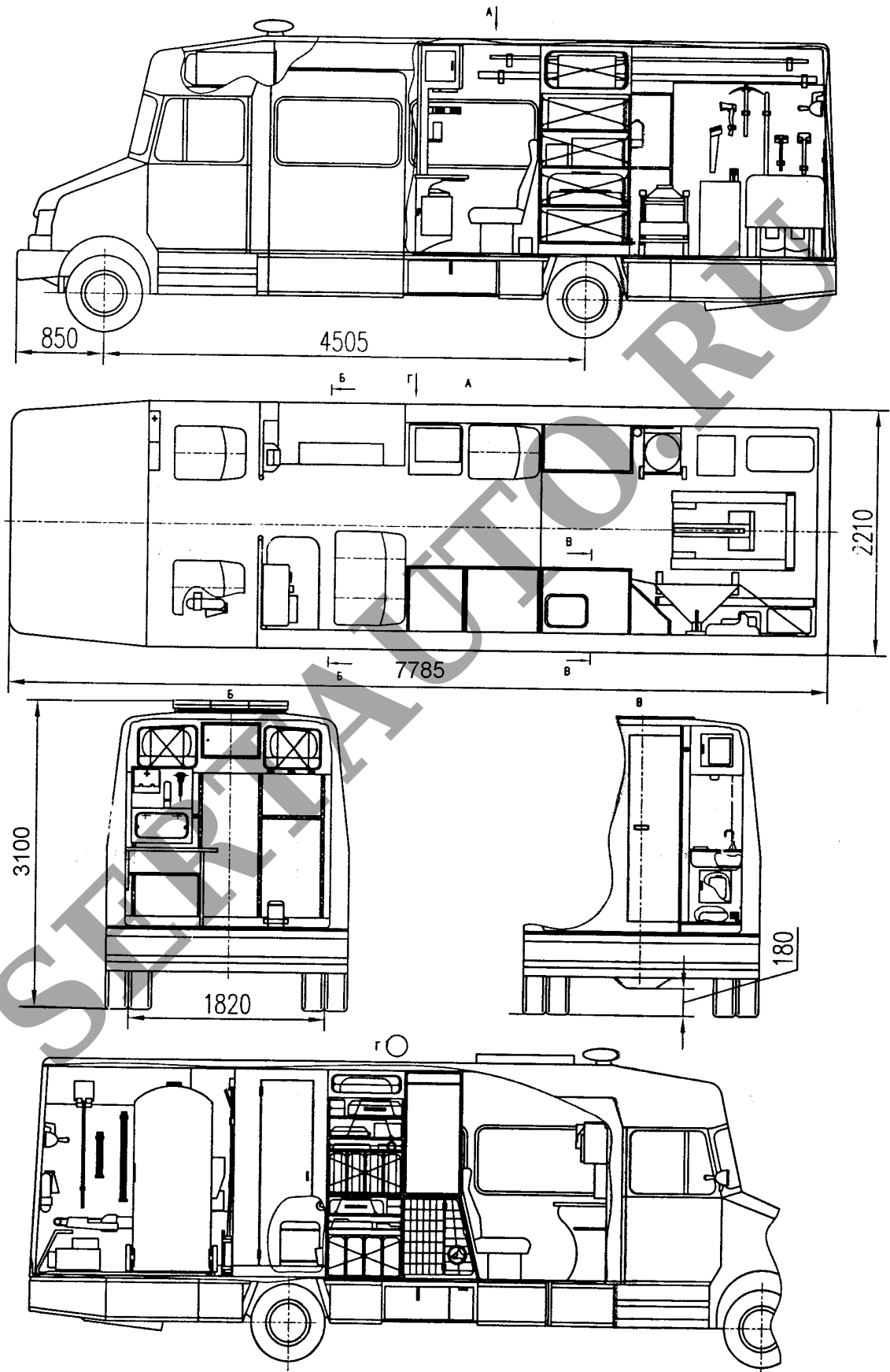
Рис. 1. Автомобиль специальный для поиска и обезвреживания взрывоопасных объектов модели 29622 (29622-0000010) / ПКО "АРАКС" на базе ЗИЛ 325000.
