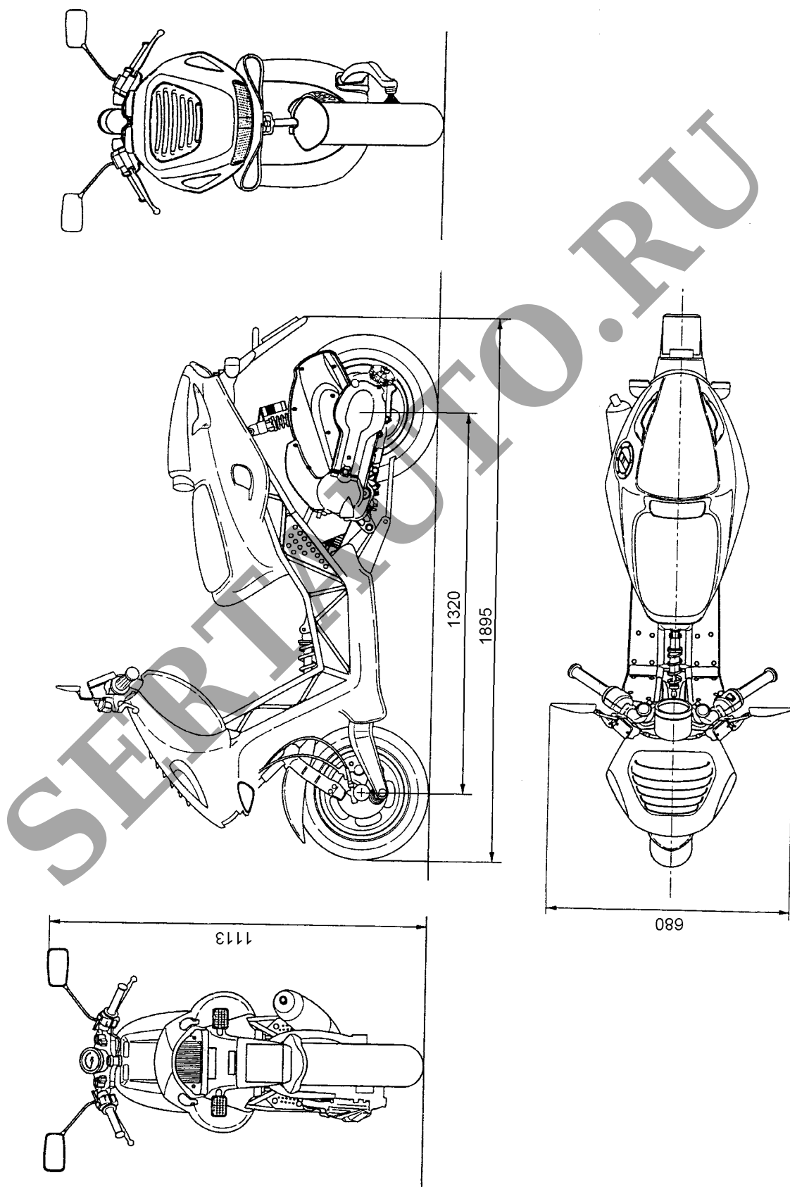
Рис.1. Мотоцикл ITALJET модели DR58 (DRAGSTER 180)
