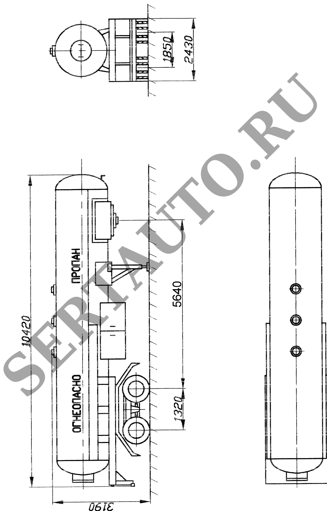
Рис.1. Полуприцеп-цистерна модели 96111 (96111-0000010)
