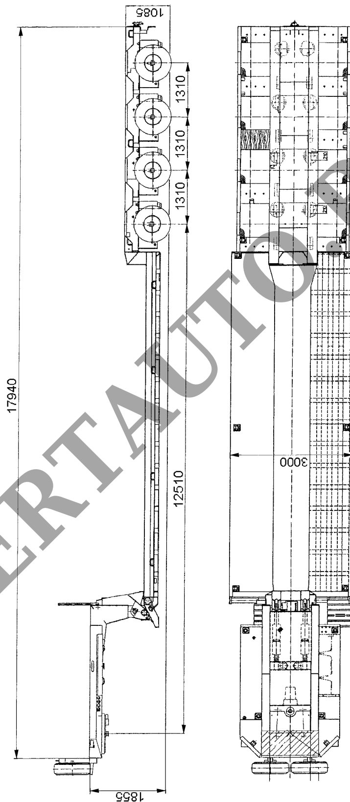
Рис.1. Полуприцеп GOLDHOFER модели STZ –VL4
