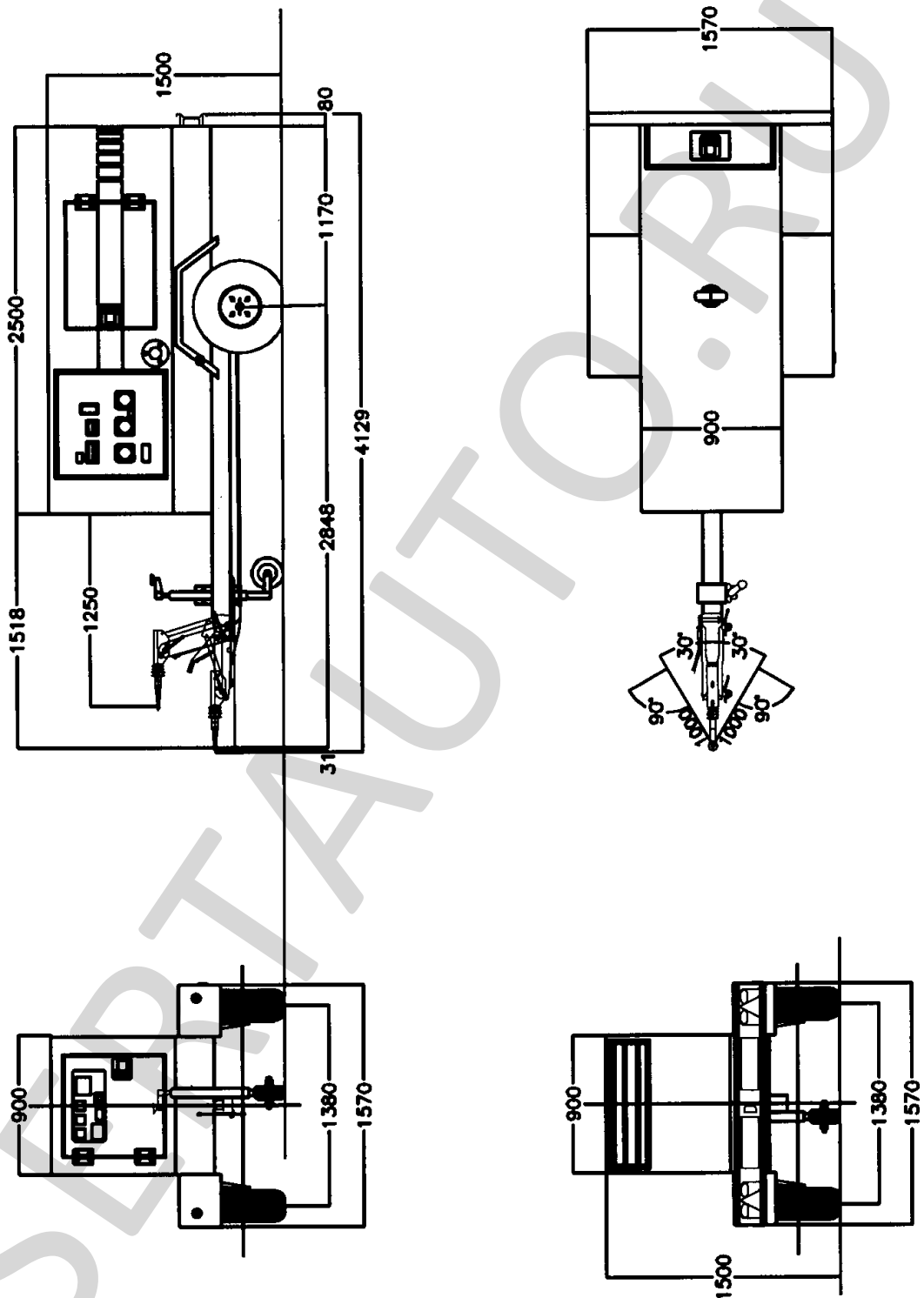
Рис. 1. Прицеп специальный с дизель-генераторной установкой Green Power модели GPG15
