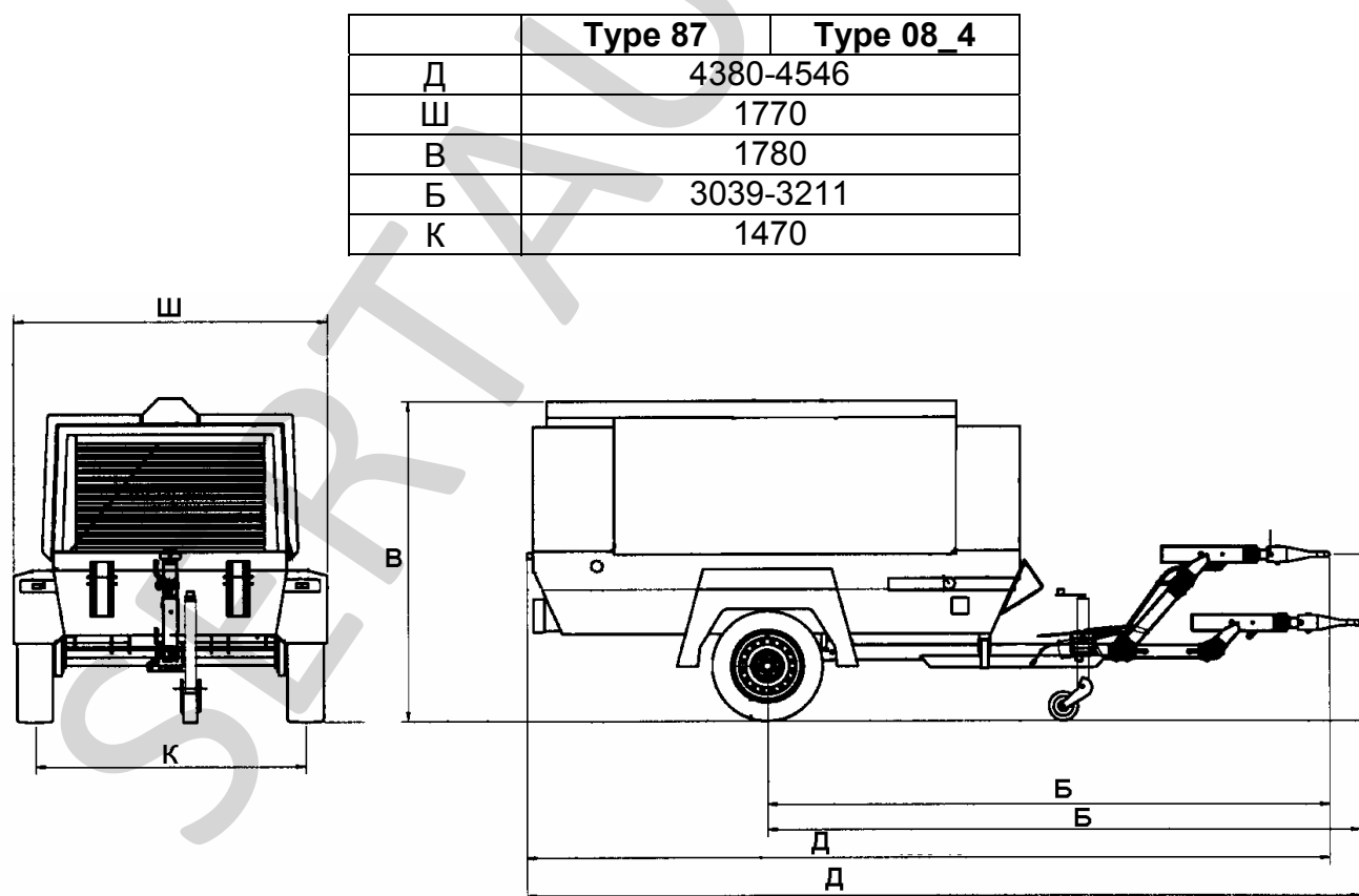
Рис. 1. Прицеп специальный марки IRMER + ELZE моделей IRMAIR 3.5, IRMAIR 4.0, IRMAIR 4.0G, IRMAIR 5.5 (Type 848586); IRMAIR 8.0, IRMAIR 11.0 (Type 87); IRMAIR 11-12H (Type 08_4).
