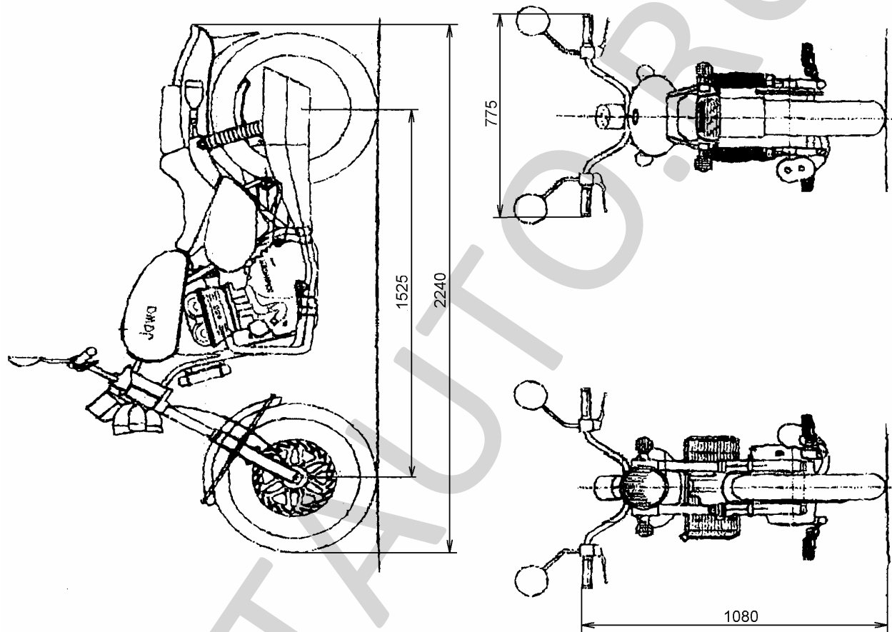
Рис.1. Мотоцикл JAWA 650 модели 836 0 (Classic)
