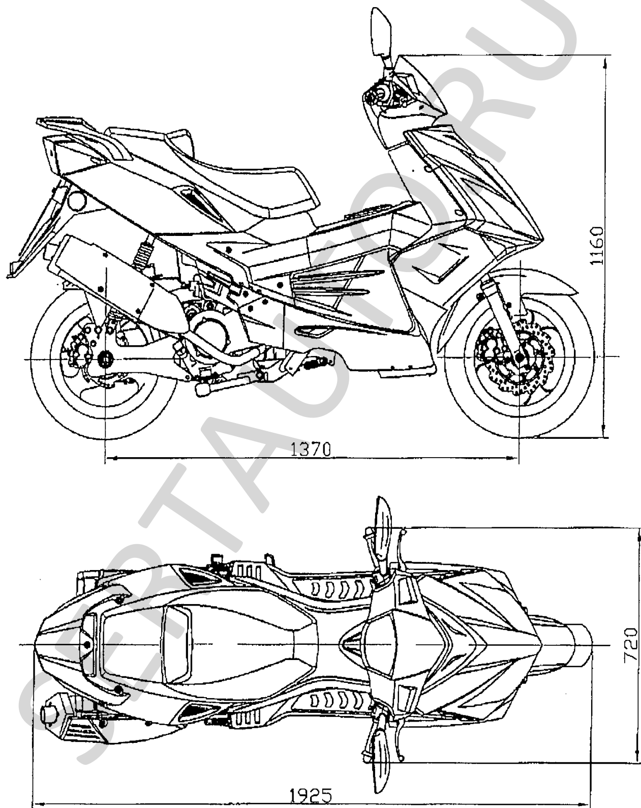
Рис. 1. Мотоцикл HUONIAO; HAOtian модели HN 125T-9 (HN 125T-9, HT 125T-9)
