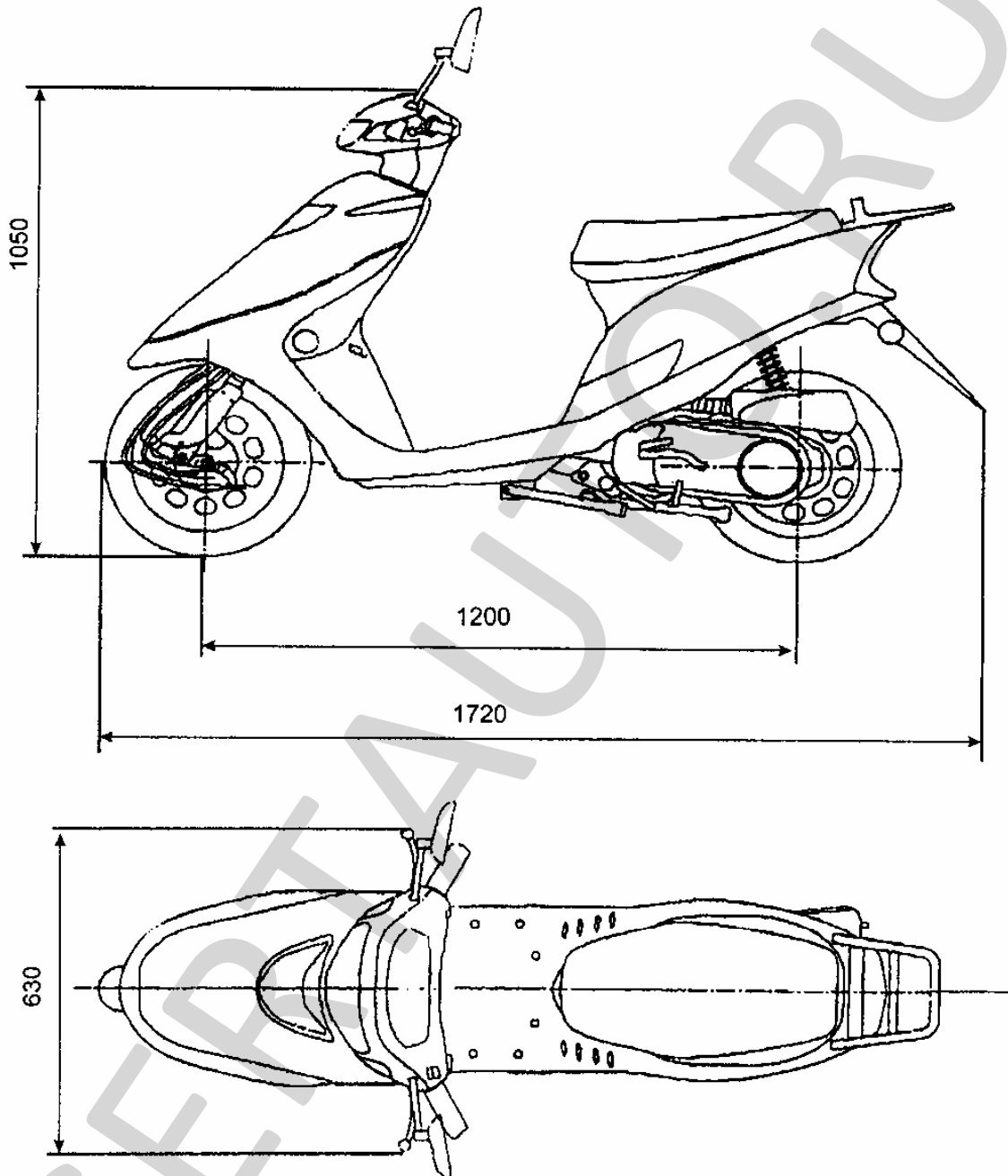
Общий вид мотороллера LF50QT-4
