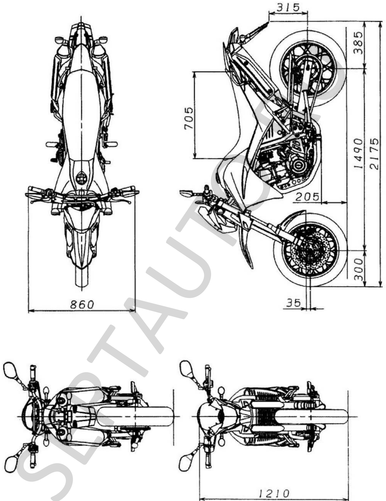
Рис. 2. Мотоцикл YAMAHA, тип DM01, вариант исполнения I/v, I/vi, I/vii (XT660 X).
