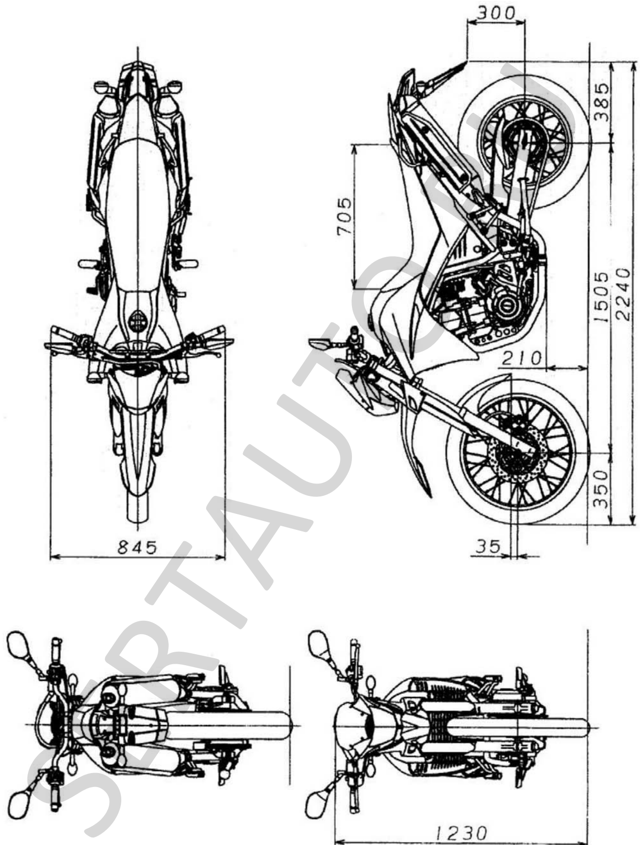
Рис. 1. Мотоцикл YAMAHA, тип DM01, вариант исполнения I/I, I/ii, I/iii (XT660 R).
