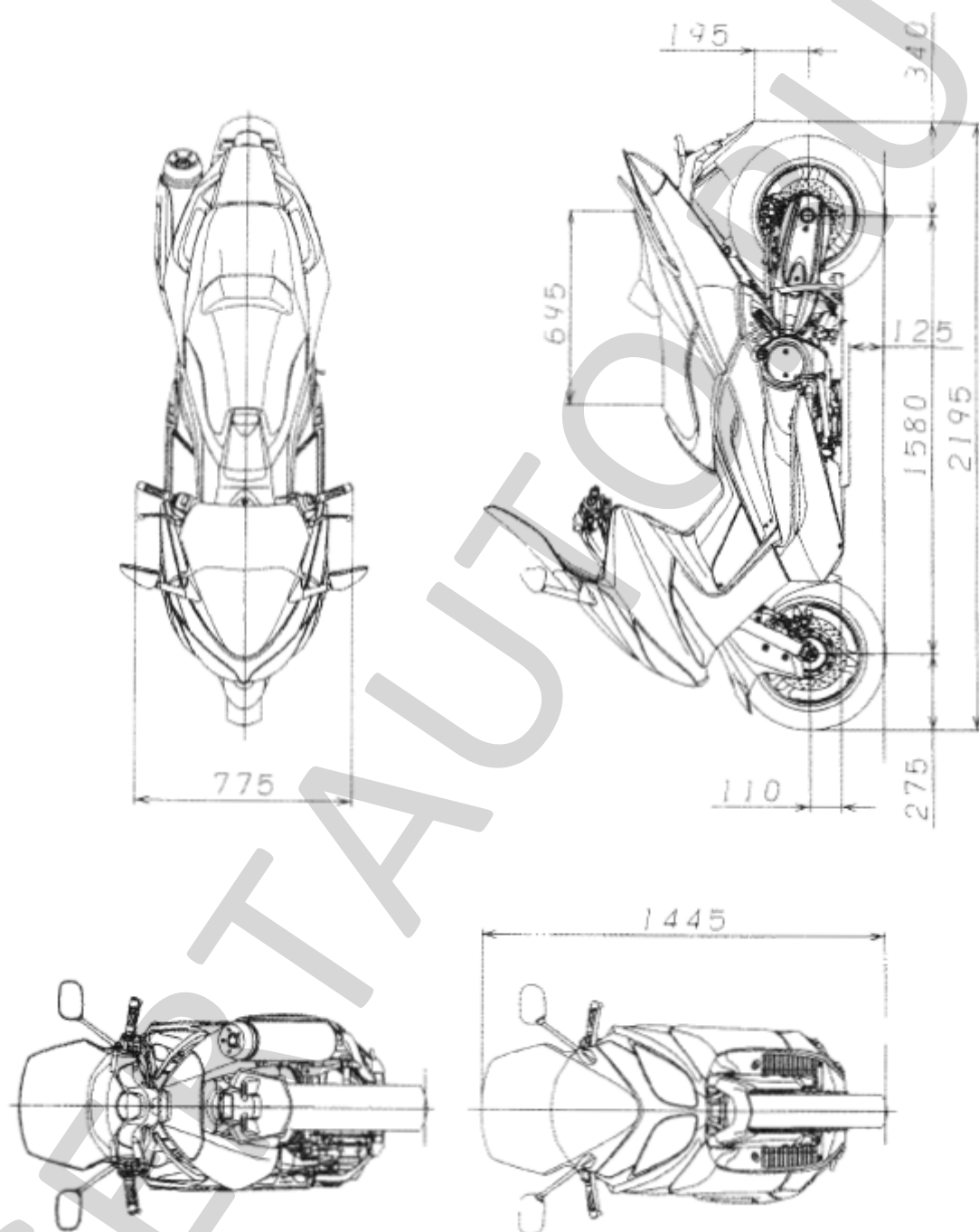
Рис. 1. Мотоцикл YAMAHA модели SJ06 (XP 500 или XP500A).
