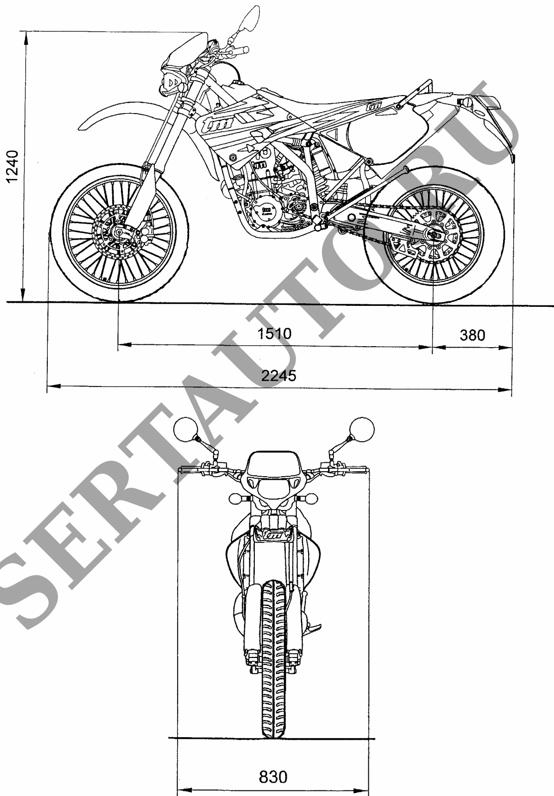
Рис. 2. Мотоцикл TM RACING 530 (F 00) моделей SUPERMOTARD SMR 530 F ES, SMM 530 F ES Black Dream
