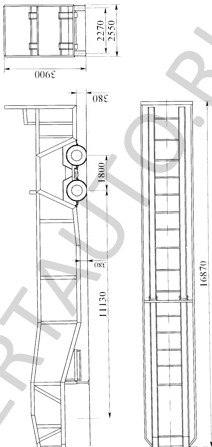
Рис. 1. Полуприцеп - автовоз модели 9963E0
