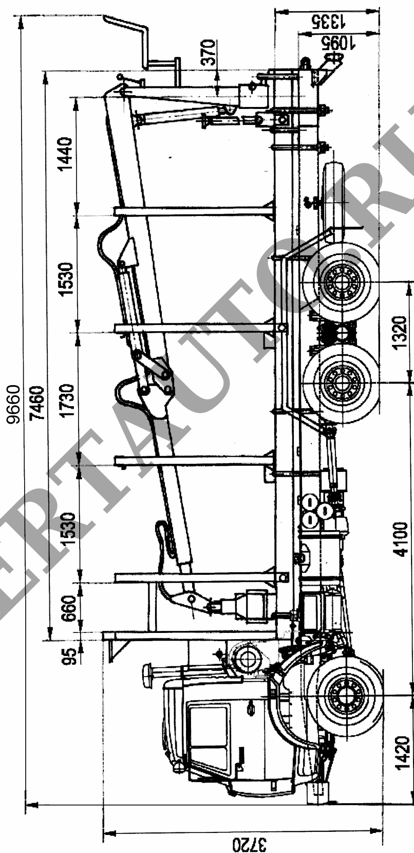
Рис. 2. Автомобиль специальный - сортиментовоз модели 54362В
