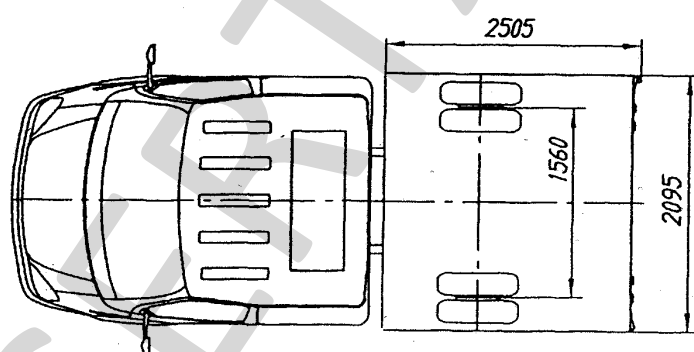
Автомобили 2704А5, 2704В5
