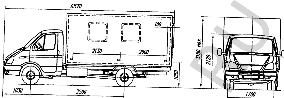
Автомобили 2704А3, 2704В3, 2704D3, 2704F3
