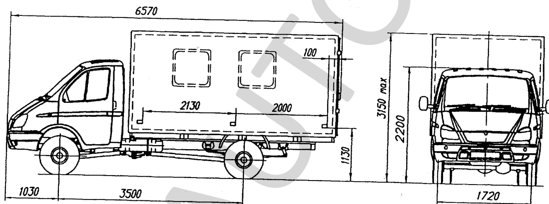
Автомобили 2704А3, 2704В3, 2704D3, 2704F3
