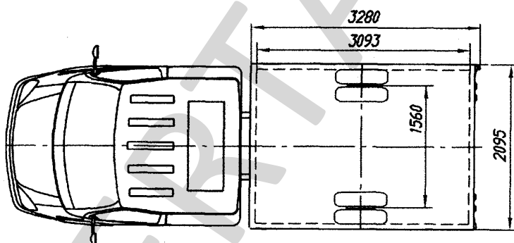
Автомобили 2704А7, 2704В7
