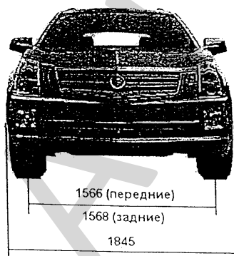
Автомобиль Cadillac GMT 265 (6EВ26 SRX)
