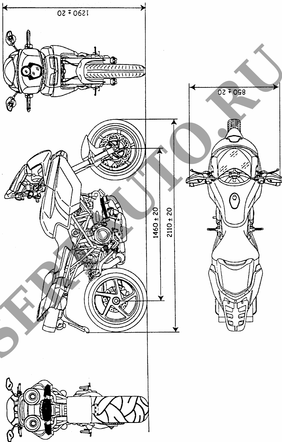
Рис. 1. Мотоцикл DUCATI моделей MTS 1000 (MTS 1000 DS), MTS 1000S (MTS 1000 SDS) без кофров
