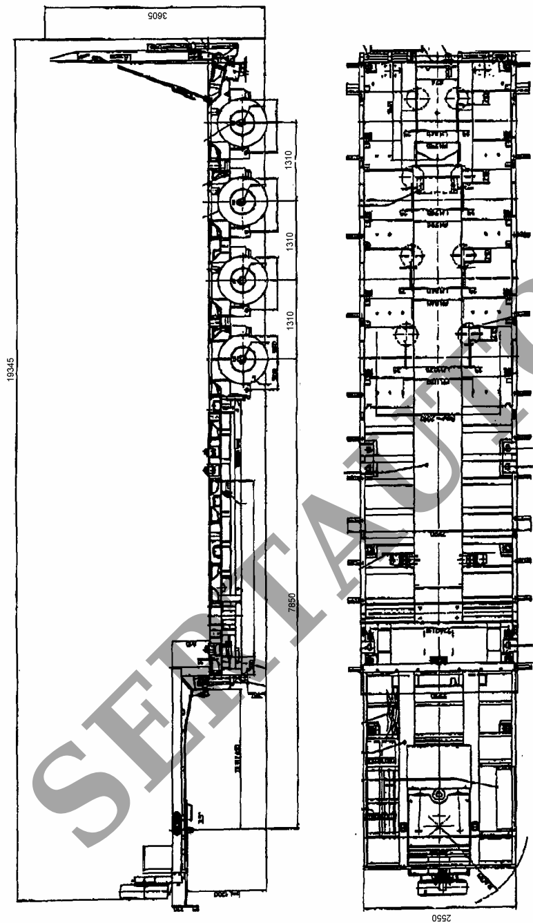
Рис.1. Полуприцеп GOLDHOFER модели STZ – L4 – 58/40A
