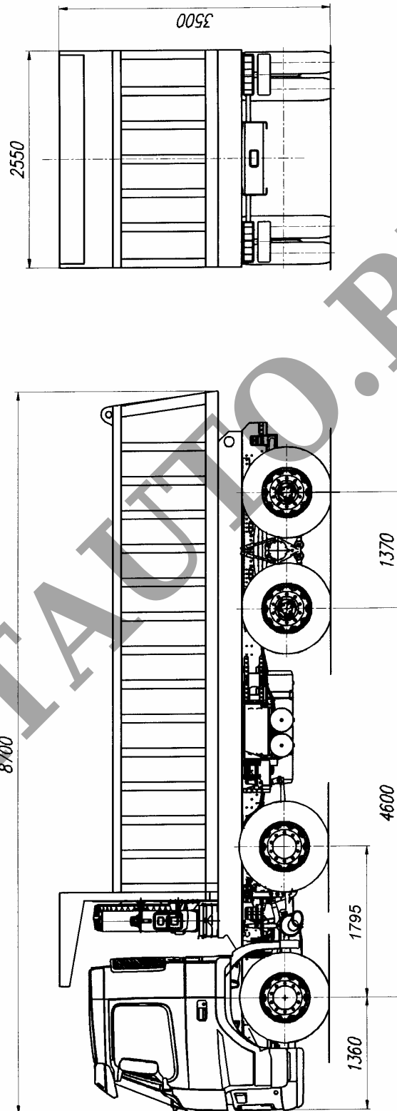
Рис.1. Автомобиль-самосвал модели 6730VK
