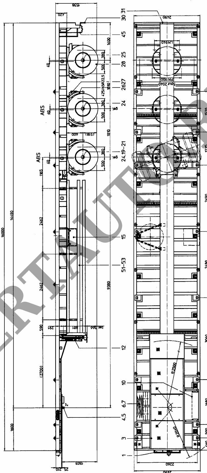
Рис.1. Полуприцеп GOLDHOFER модели SPZ – DL3 – 36/80
