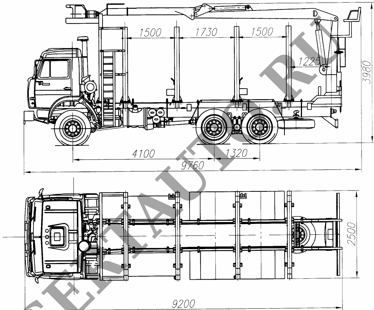
Рис.2. Автомобиль сортиментовоз модели 63792В (6379-000010-22) / КСМ3-53228 на шасси КамАЗ 53228
