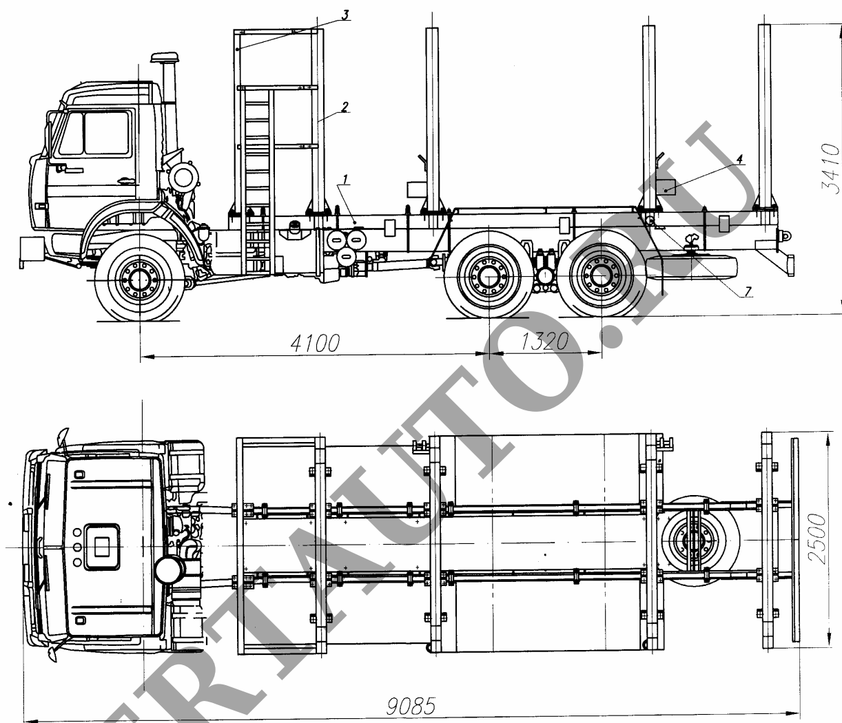
Рис. 1. Автомобиль сортиментовоз модели 63791В (6379-0000010-21) / КС-53228 на шасси КамАЗ 53228
