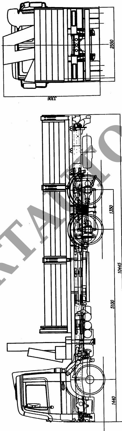
Рис. 1. Автомобиль грузовой бортовой с краном манипулятором модели 6827МК (6827-000010).
