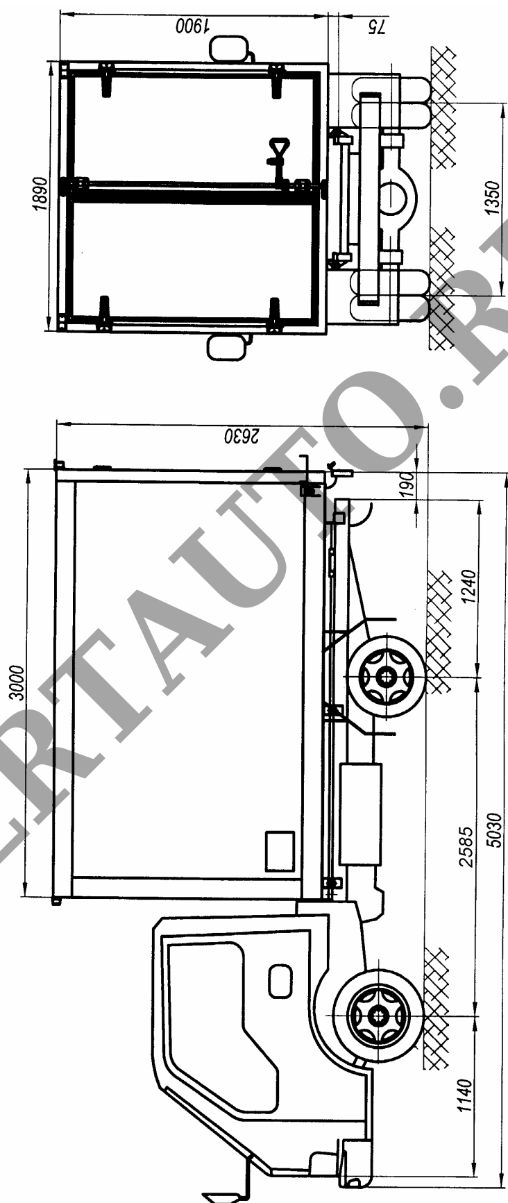
Рис.1. Автомобиль – фургон модели 47668А (47668-000010)
