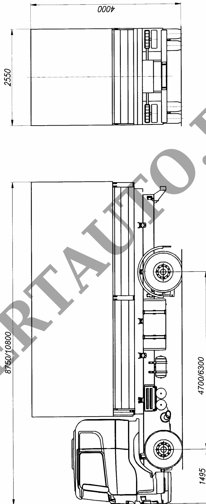
Рис.2. Автомобиль моделей 6730CR , 6730CE / 6730CD
