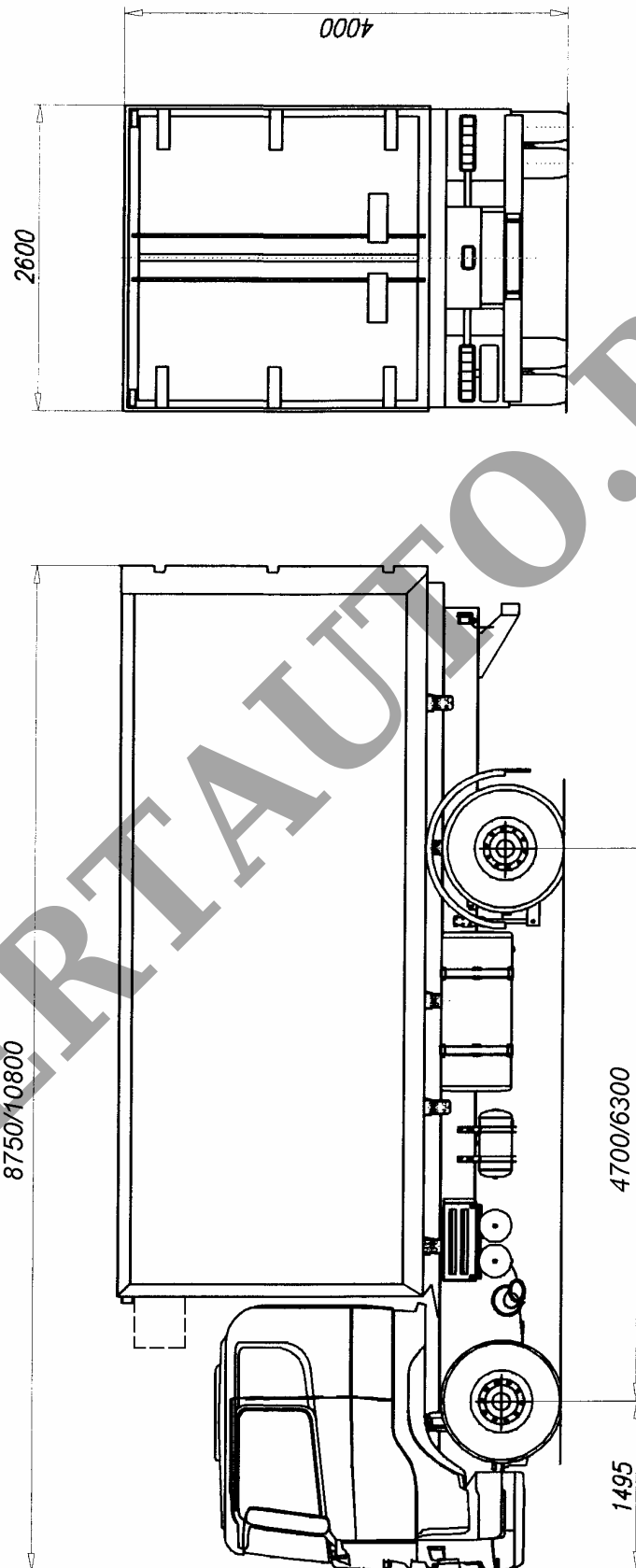
Рис.1. Автомобиль – фургон моделей 6730CA , 6730CF/ 6730CB
