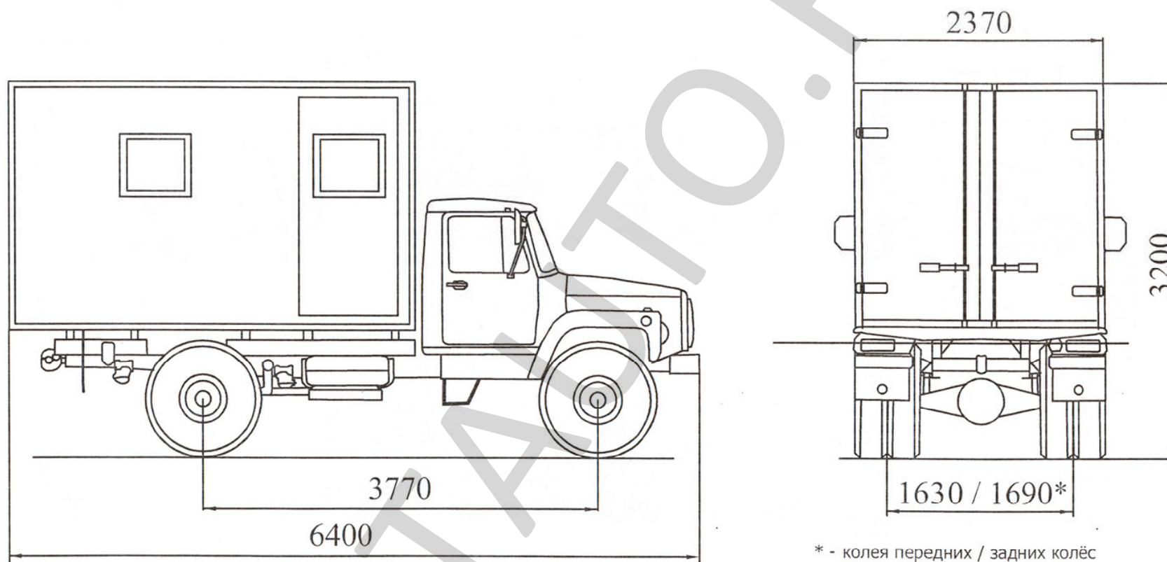
Автомобили-мастерские мод. 27901-0000010-23 (шасси ГАЗ-3309)
