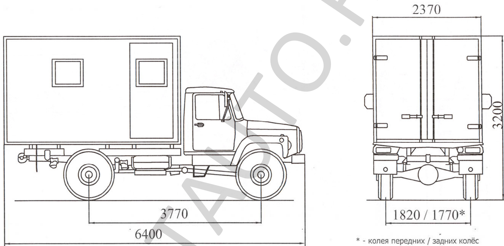
Автомобили-мастерские мод. 27901-0000010-13 (шасси ГАЗ-3308)
