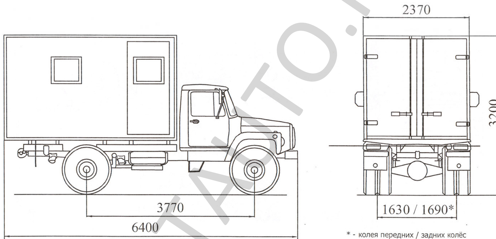
Автомобили-мастерские мод. 27901-0000010-03 (шасси ГАЗ-3307)
