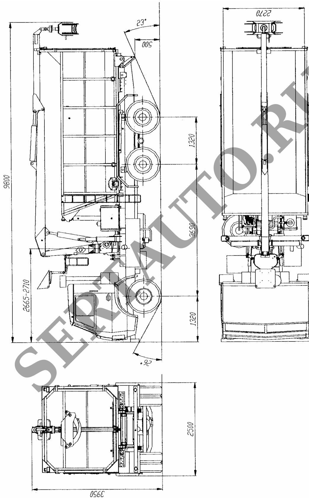
Рис. 1. Автомобиль - самосвал с краном - манипулятором модели 5872 (5872-000010)
