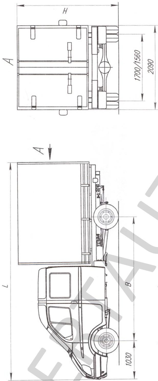
Специализированная платформа
