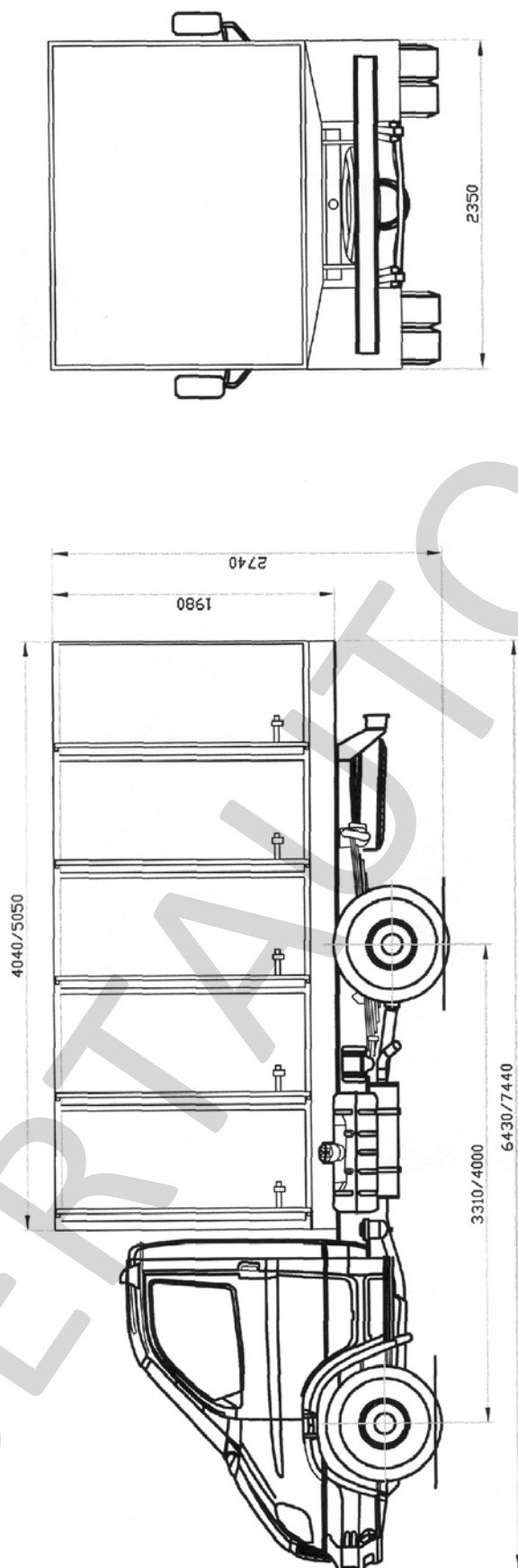
Хлебный автофургон 28182-0000010-03 на базе шасси ГАЗ-33104
