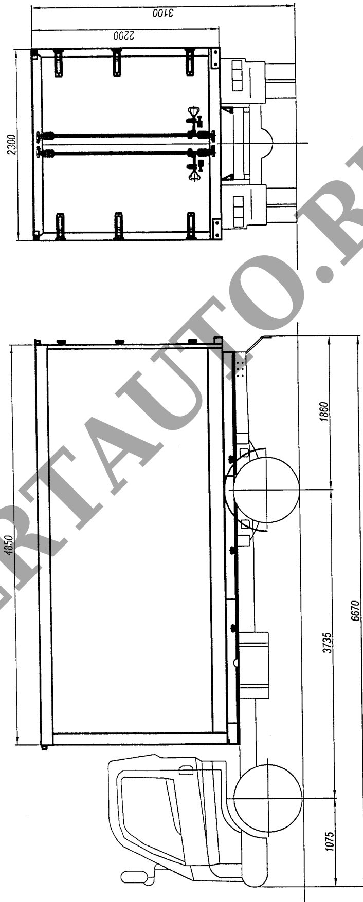
Рис.1. Автомобиль - фургон модели 47667А (47667-0000010).
