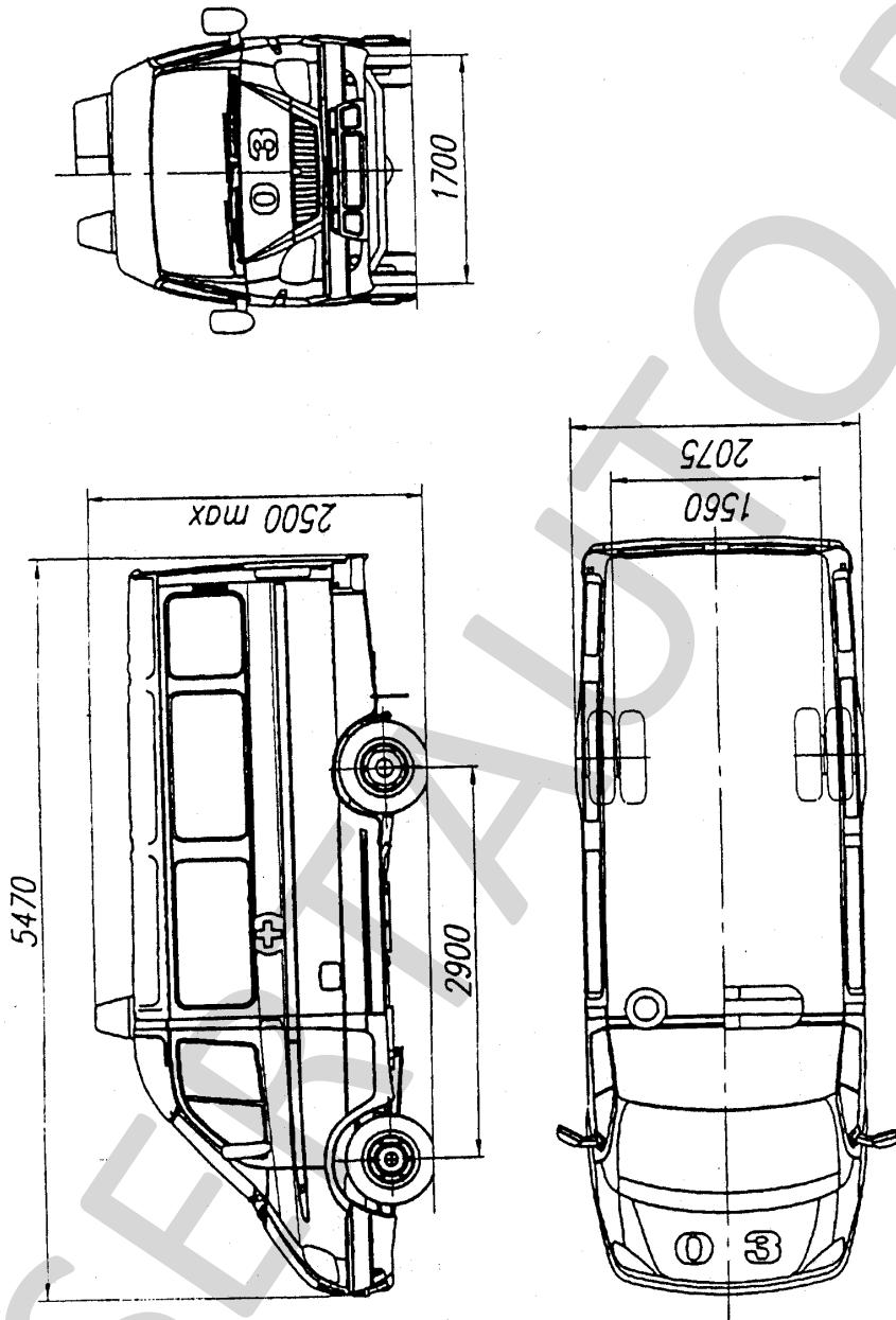
Автомобиль ГАЗ – 32214
