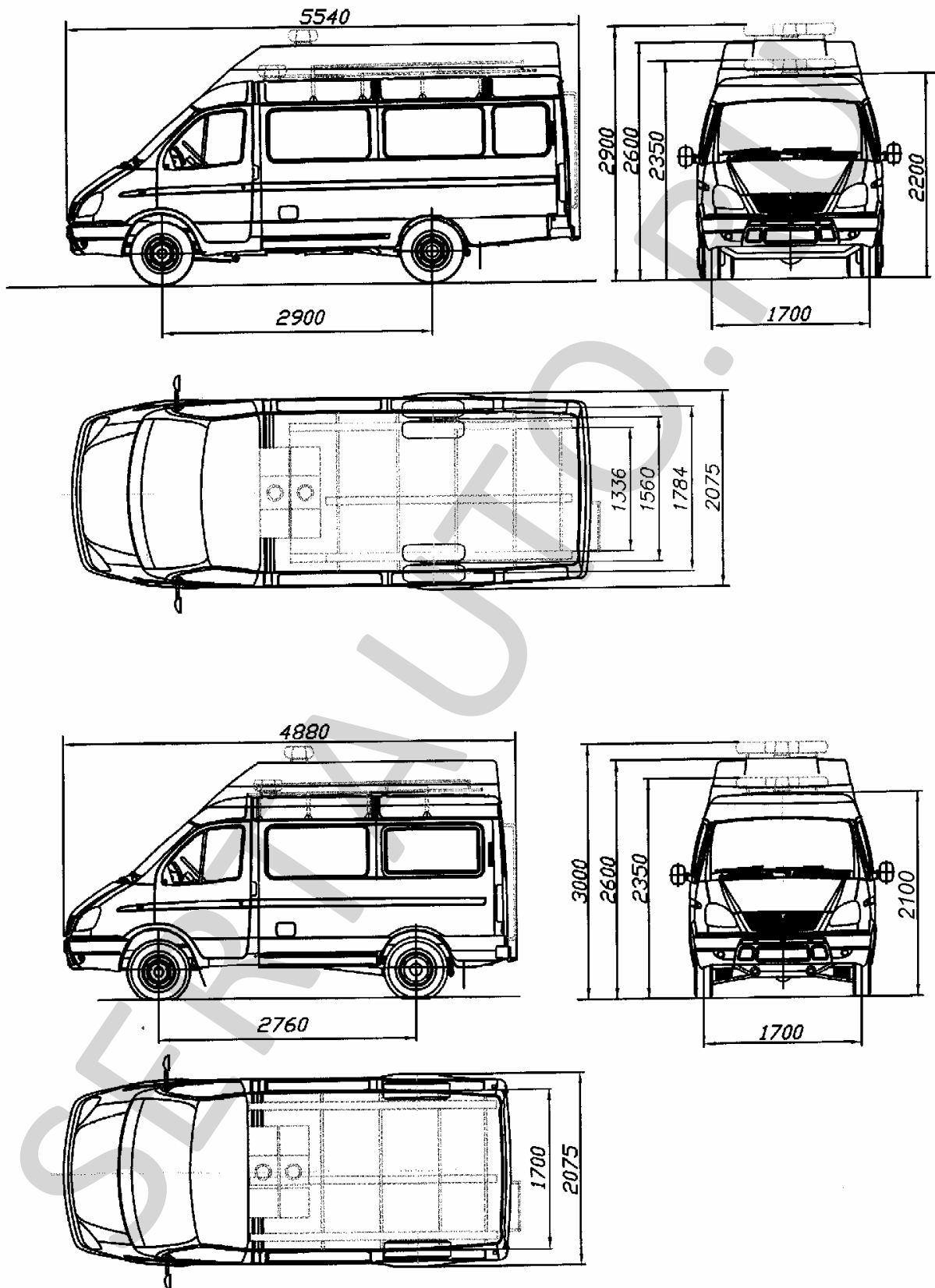
Рис. 1. Автомобиль моделей 22250В, 22250С, 22250D, 22250F, 22250G, 22252В, 22252С, 22252D, 22252F, 22252G
