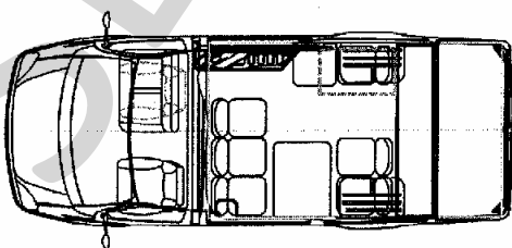
Рис. 4. Автомобиль моделей 22250В, 22250С, 22250F, 22252В, 22252С
