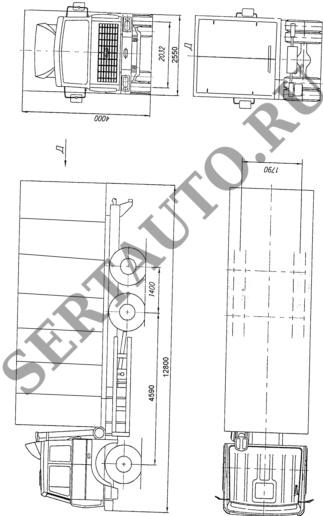
Рис.1. Автомобиль – фургон модели 5747LR (57471-0000010)
