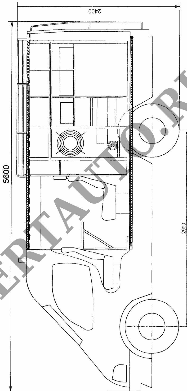
Рис.1. Автомобиль-мастерская модели 29620S (МДМ) (машина дорожного мастера)
