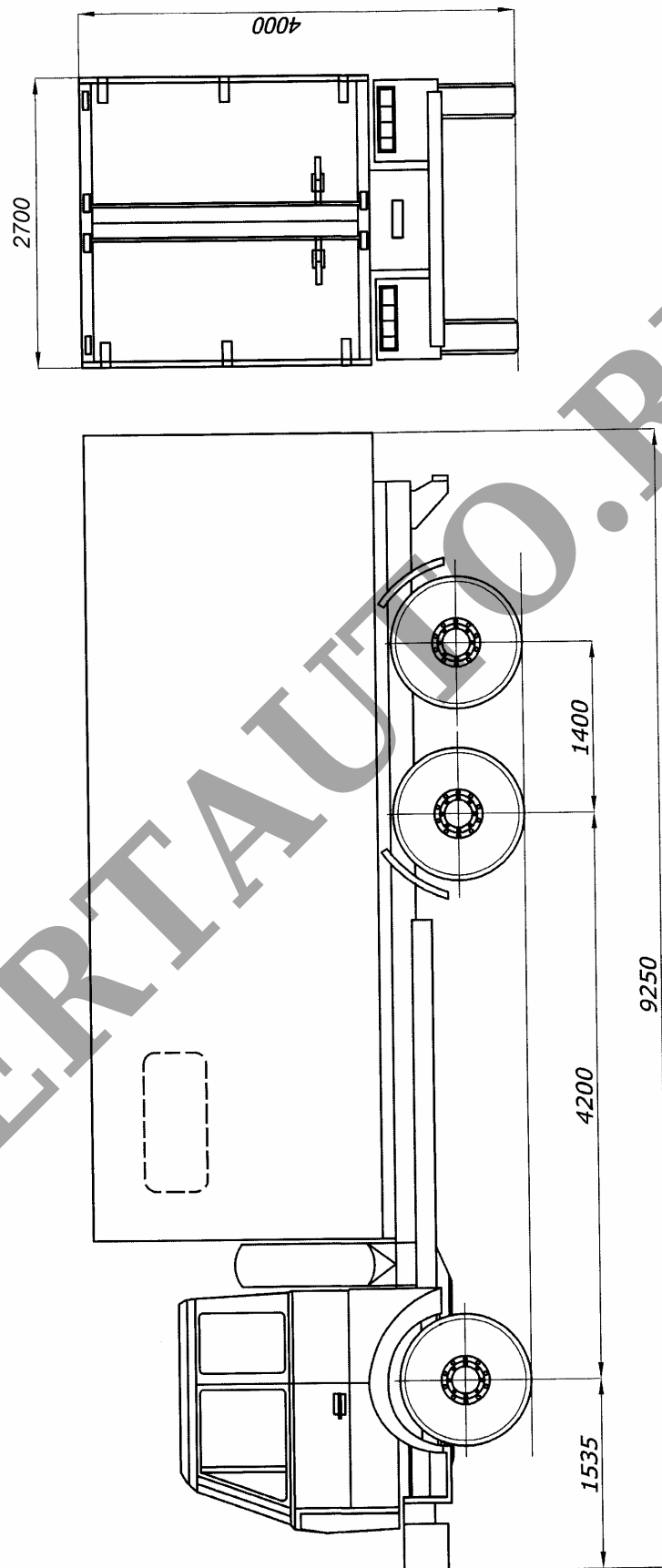
Рис 3. Автомобиль-фургон моделей 5763FR, 5763TR, автомобиль-мастерская модели 5763MR.
