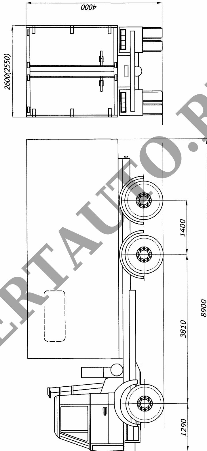
Рис.1 Автомобиль-фургон моделей 5763FC, 5763TC, автомобиль-мастерская модели 5763MC.
