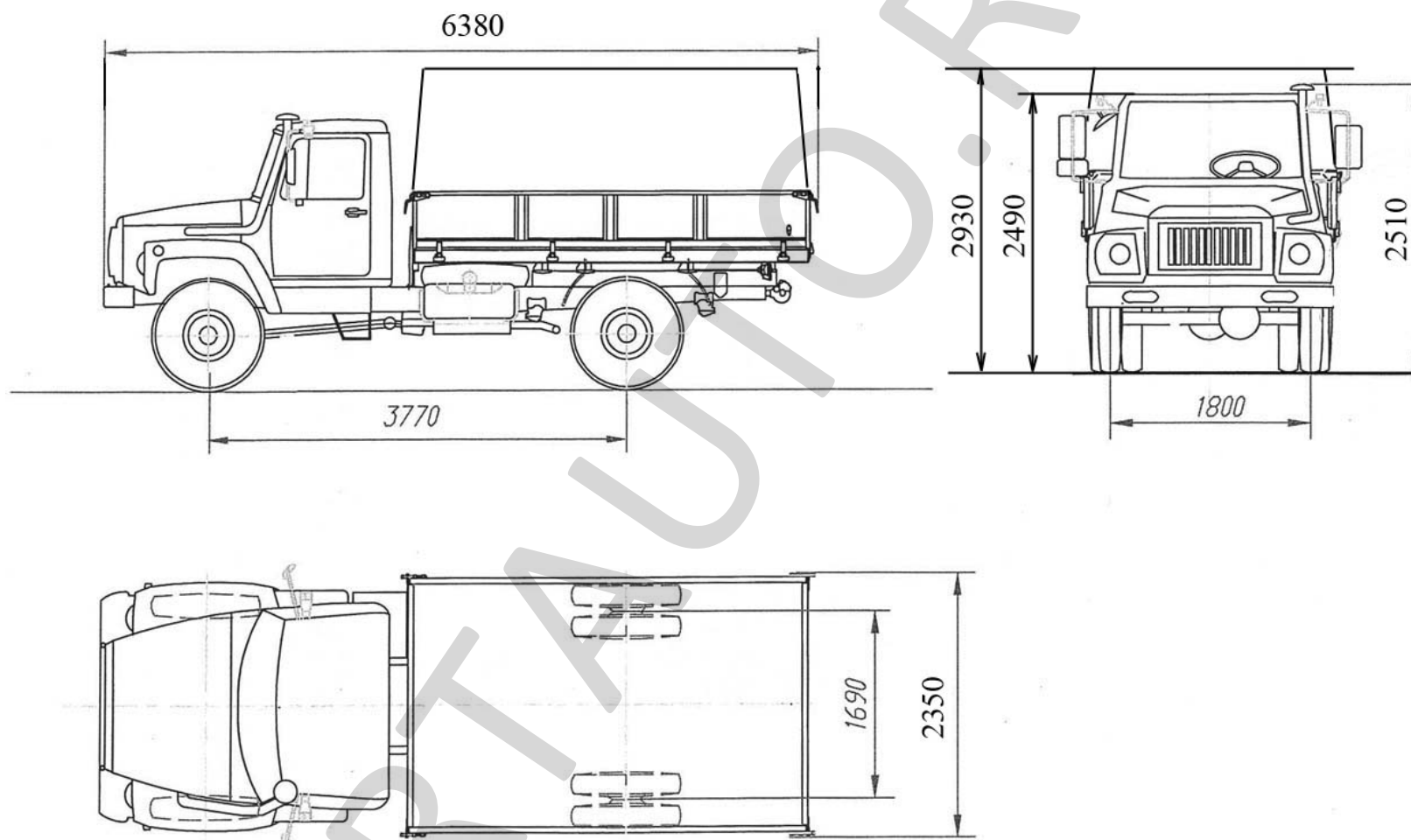
Автомобиль ГАЗ-33086
