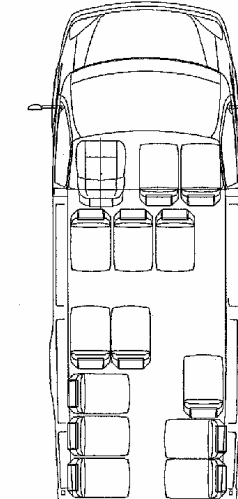
ГАЗ-322132, 322133
