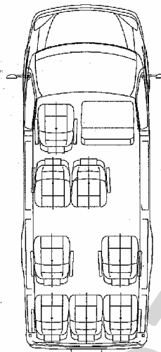
ГАЗ-3221, 32217
