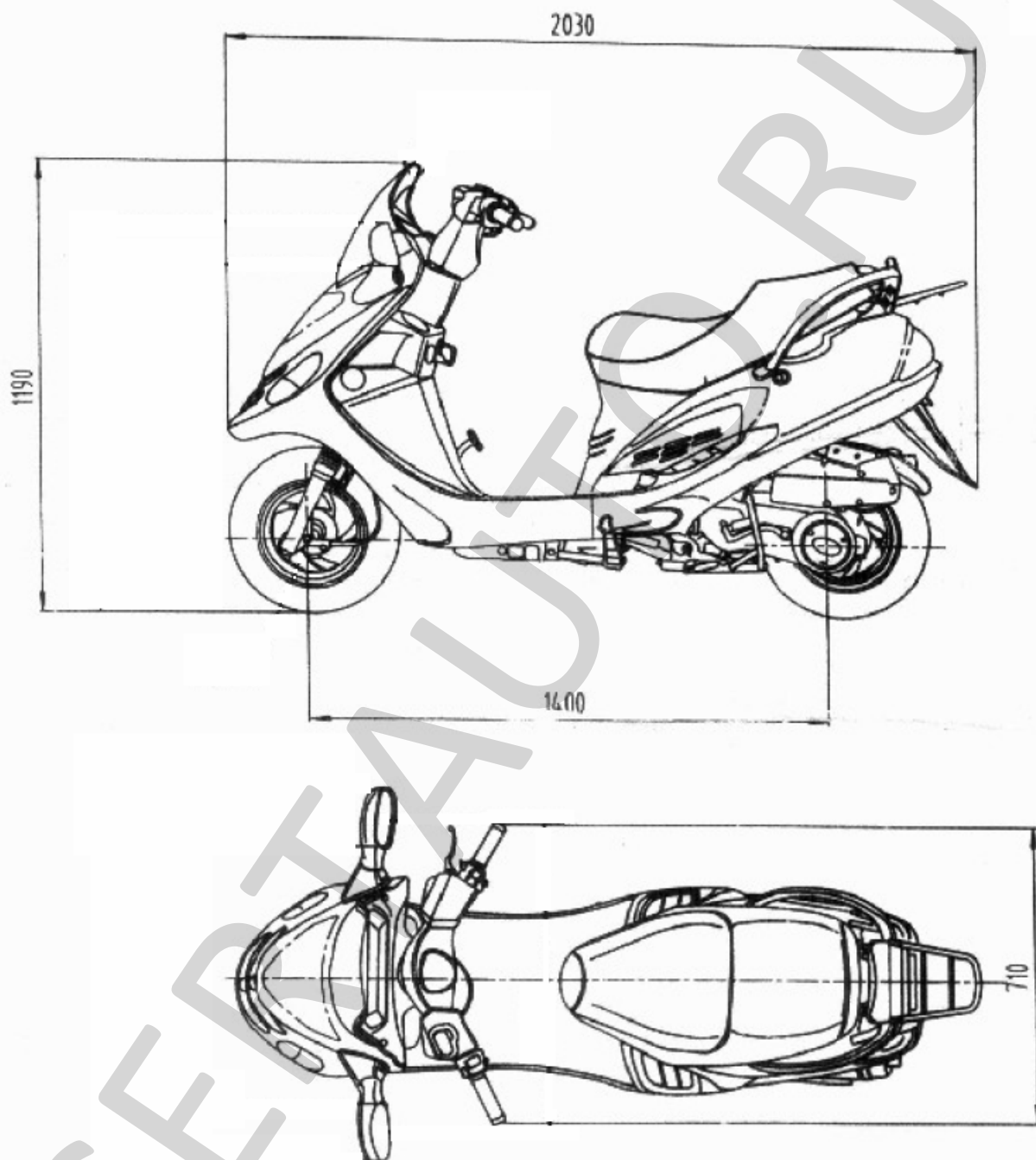
Рис. 1. Мотоцикл MEIDUO YB125T-2
