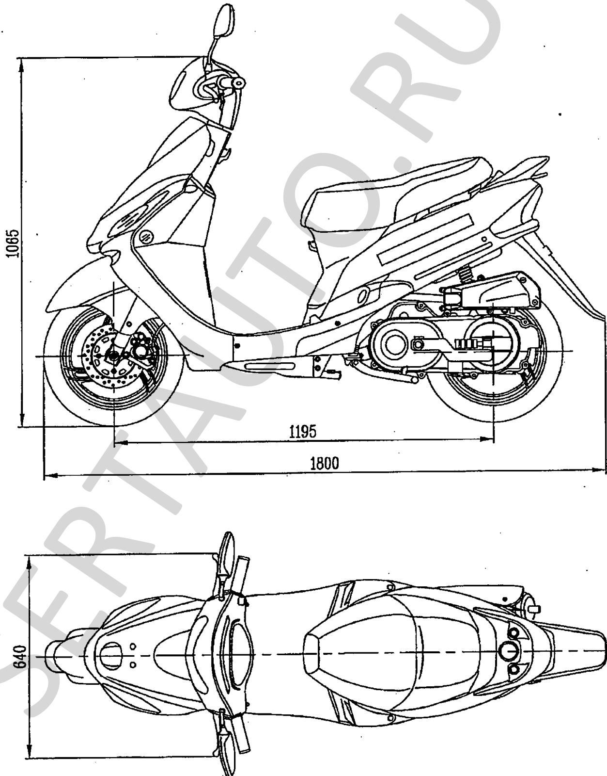
Рис. 1. Мопед HUONIAO; HAOTIAN модели HN50QT-2
