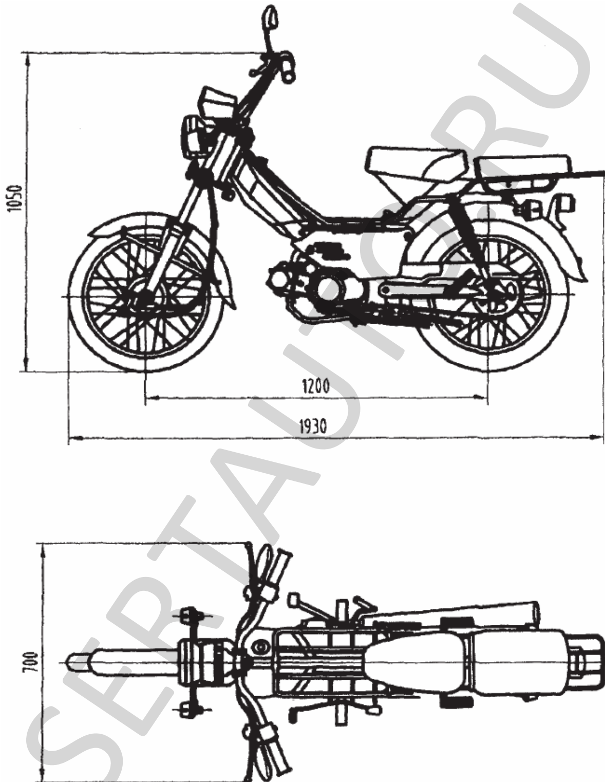
Рис. 1. Мопед YINXIANG, CHEETA, KENBO, TCB, FEKON модели YX48Q-2.
