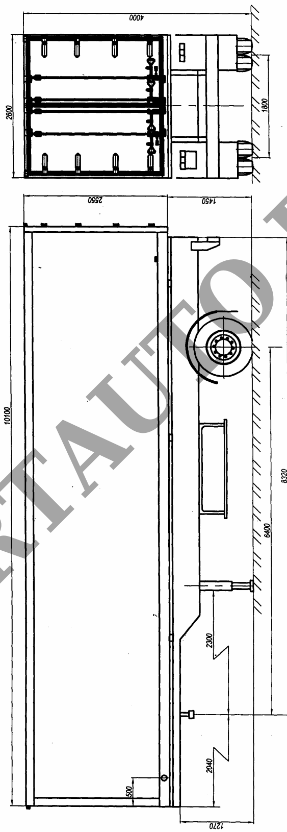
Рис. 1. Полуприцеп - фургон модели 97392А (97392-000010)
