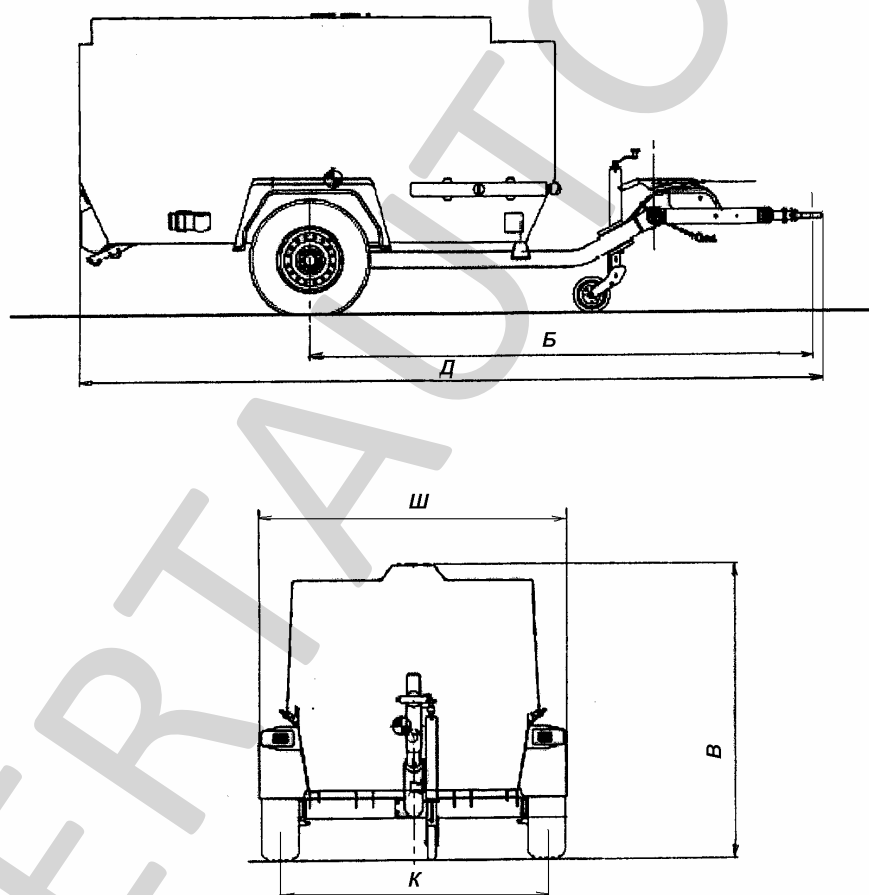
Рис. 1. Прицеп специальный ATLAS COPCO моделей, XAS 37 (Kd), XAS 47 (Kd)
