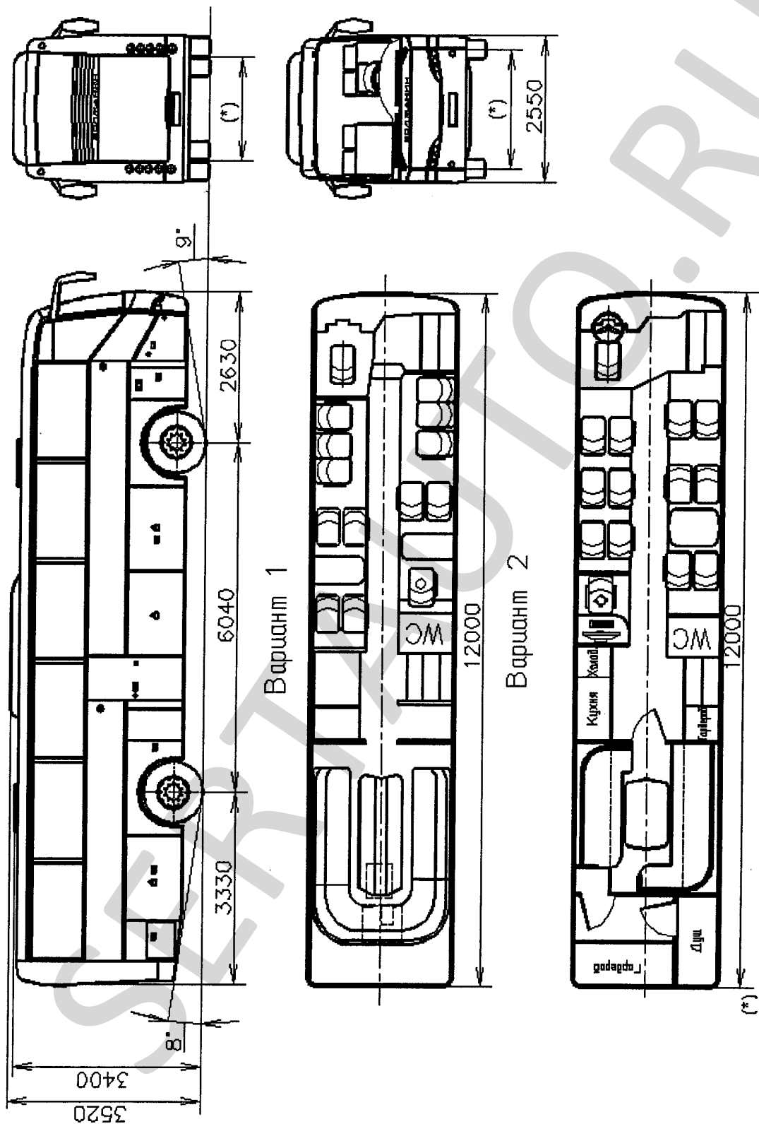
Общий вид автобуса «Волжанин 5285?-0000010-?? VIP Bus» .
