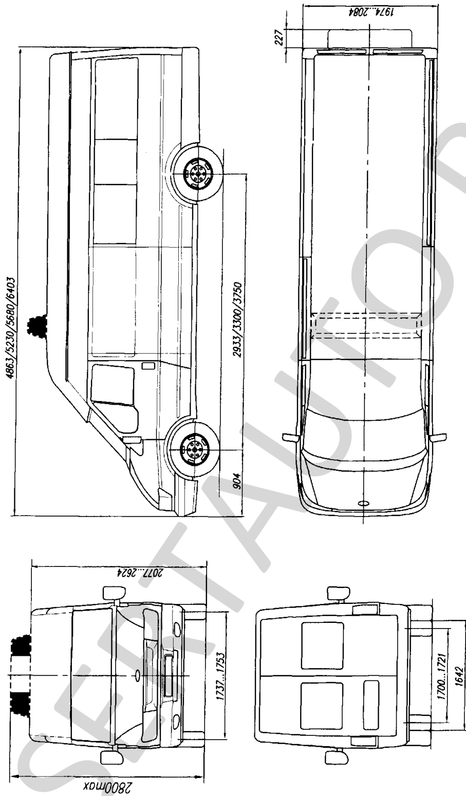
Рис. 1. Транспортные средства моделей 2227??
