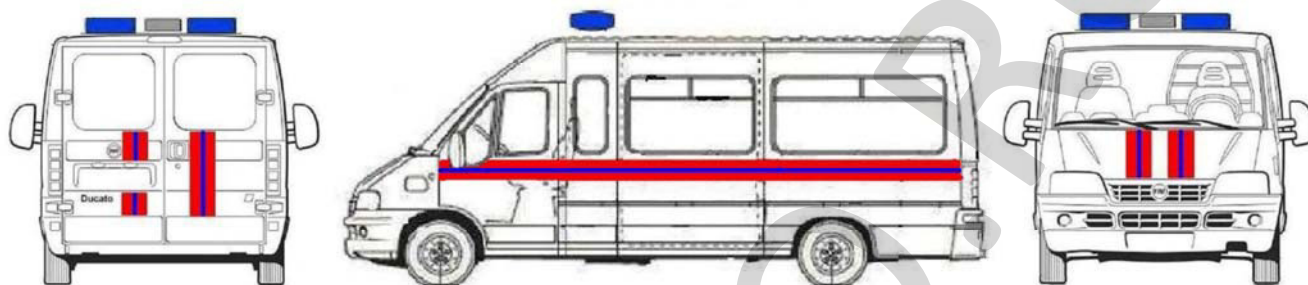
Общий вид цветографической схемы автомобиля аварийно-спасательных служб МЧС
