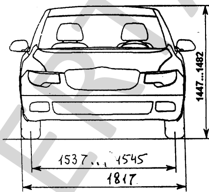
Внешний вид автомобиля категории М Skoda 3F (Superb)
