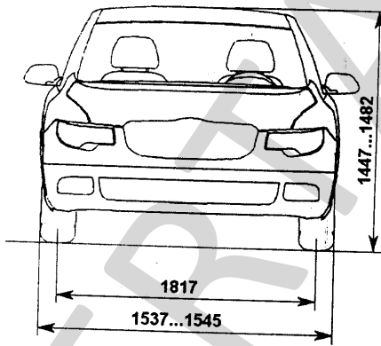
Внешний вид автомобиля категории M 1 Skoda 3T (Superb)
