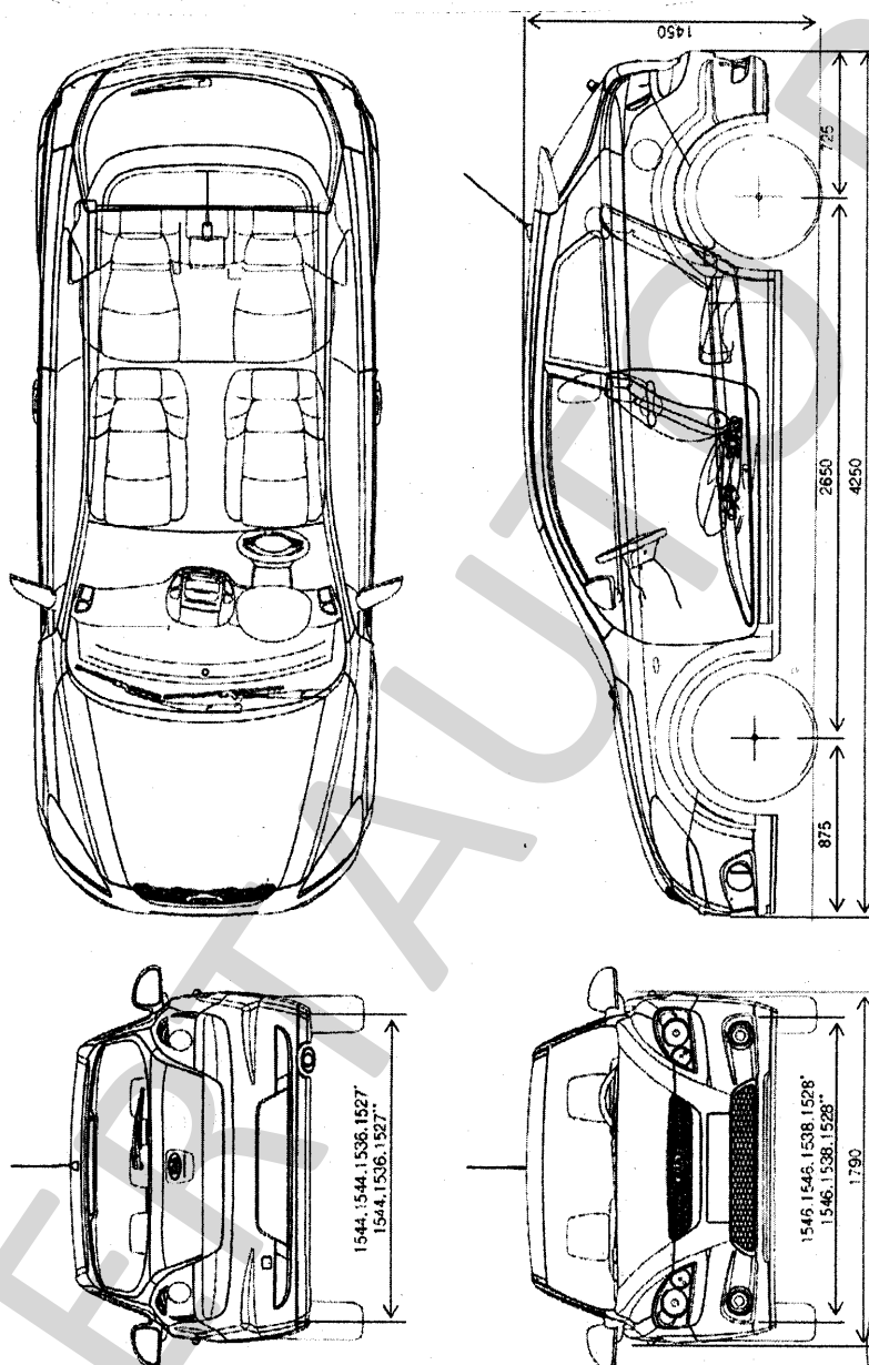
KIA ED (C'eed) хэтчбек трехдверный
