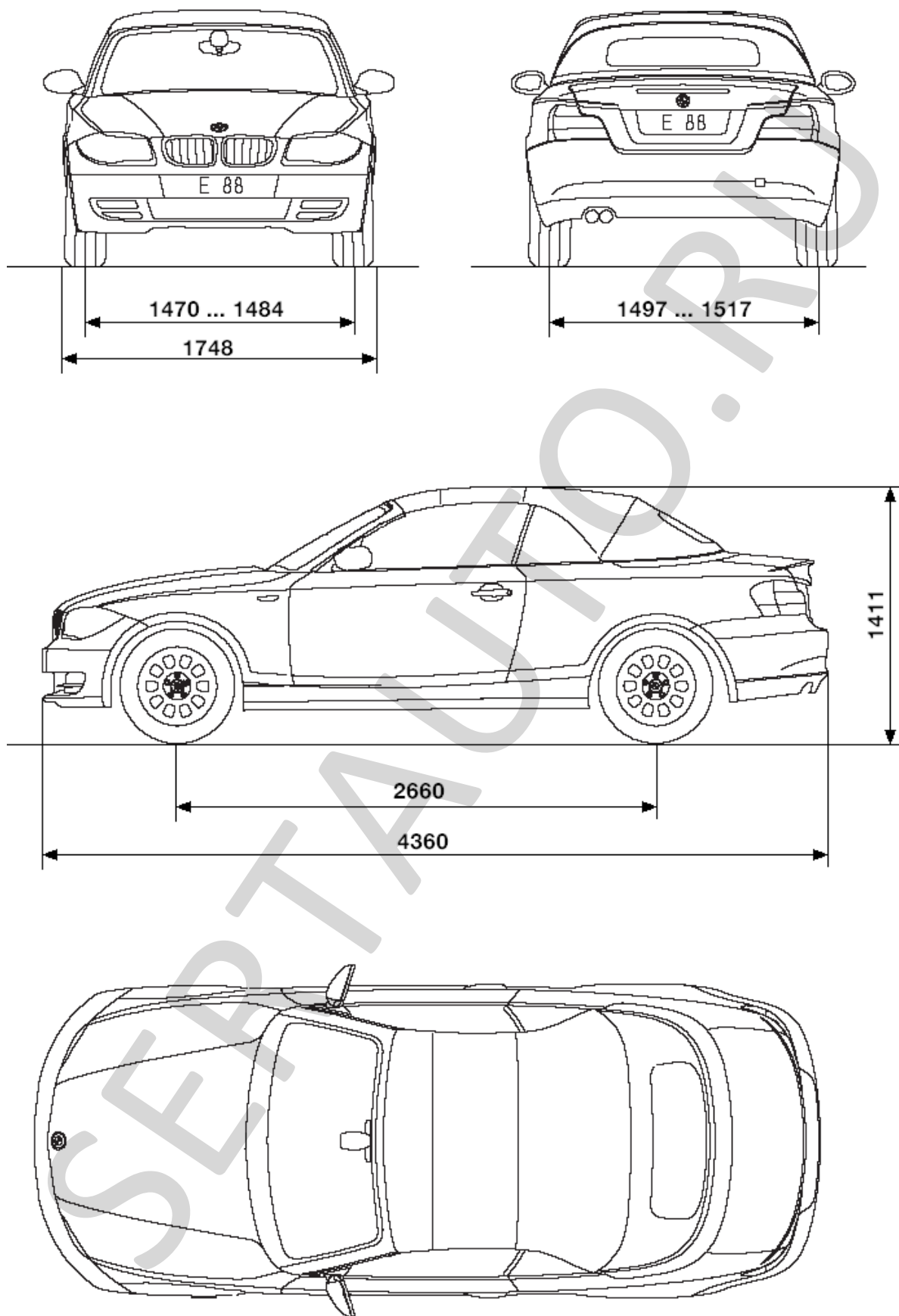
Общий вид автомобиля BMW тип 1C (кузов «Кабриолет»)
