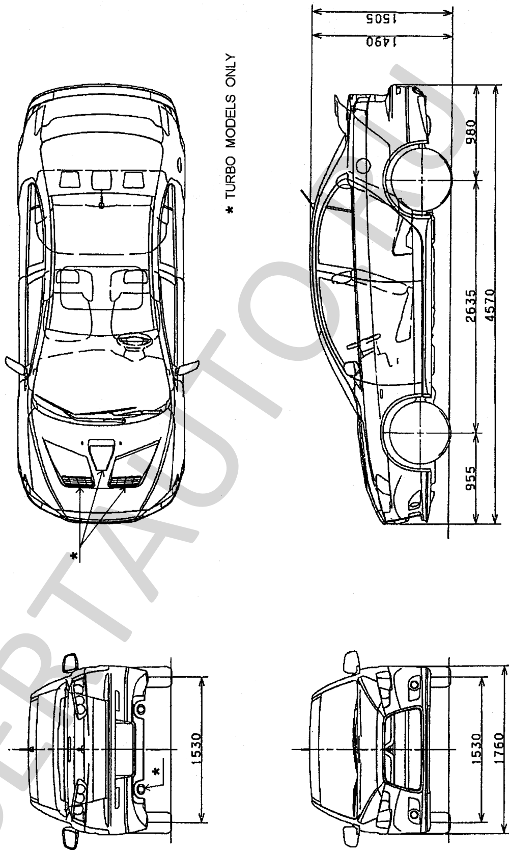
Общий вид автомобиля MITSUBISHI Lancer (CY?AS...)
