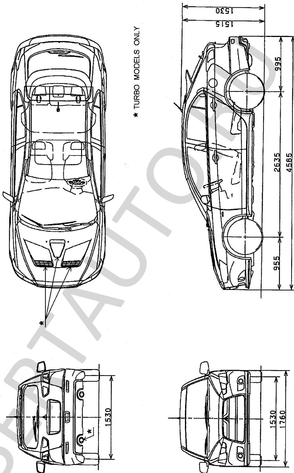
Общий вид автомобиля MITSUBISHI Lancer (CX?AL...)
